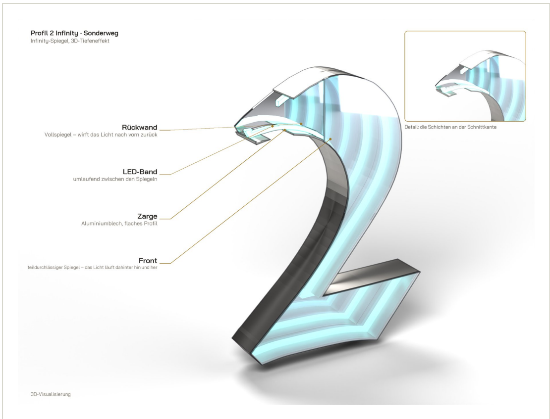
SCHNITT · PROFIL 2 INFINITY
