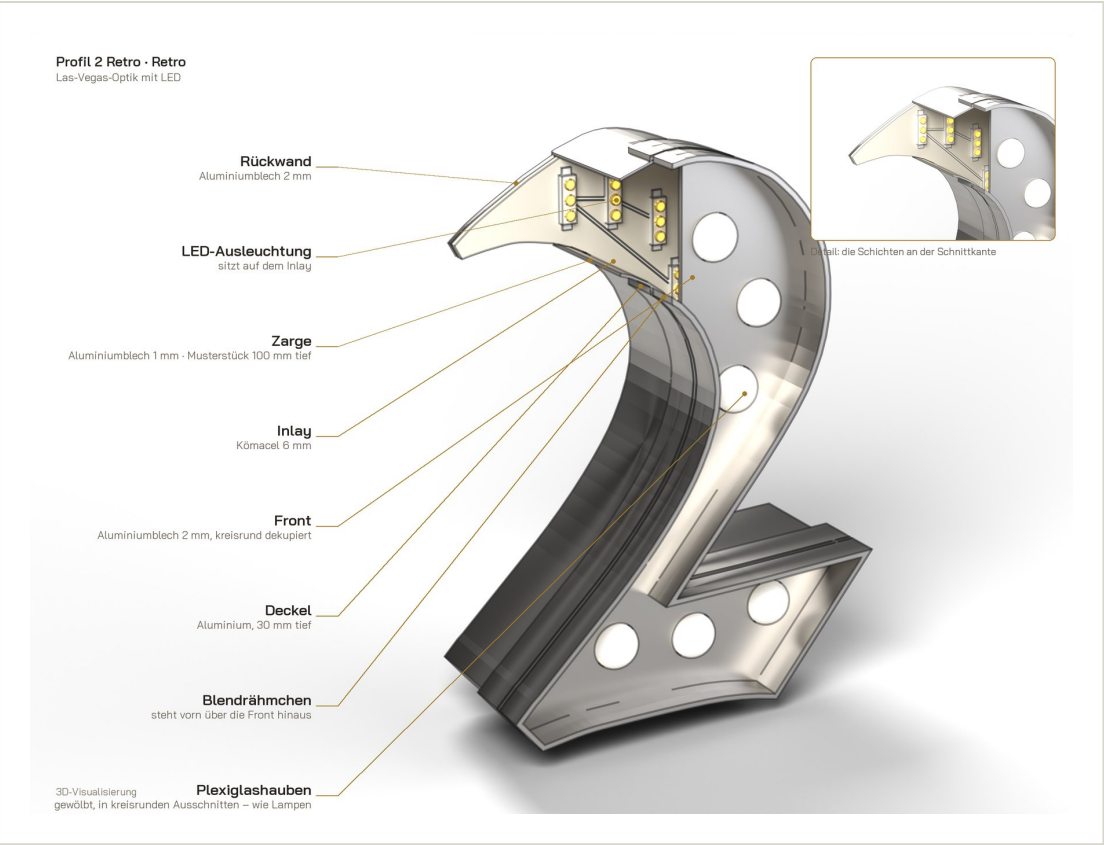
SCHNITT · PROFIL 2 RETRO
