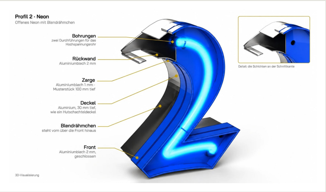
SCHNITT · PROFIL 2
