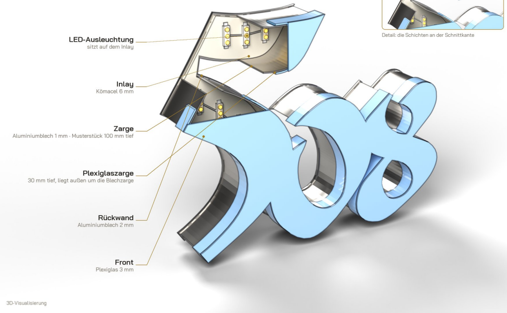
SCHNITT · PROFIL 5/08-LED
