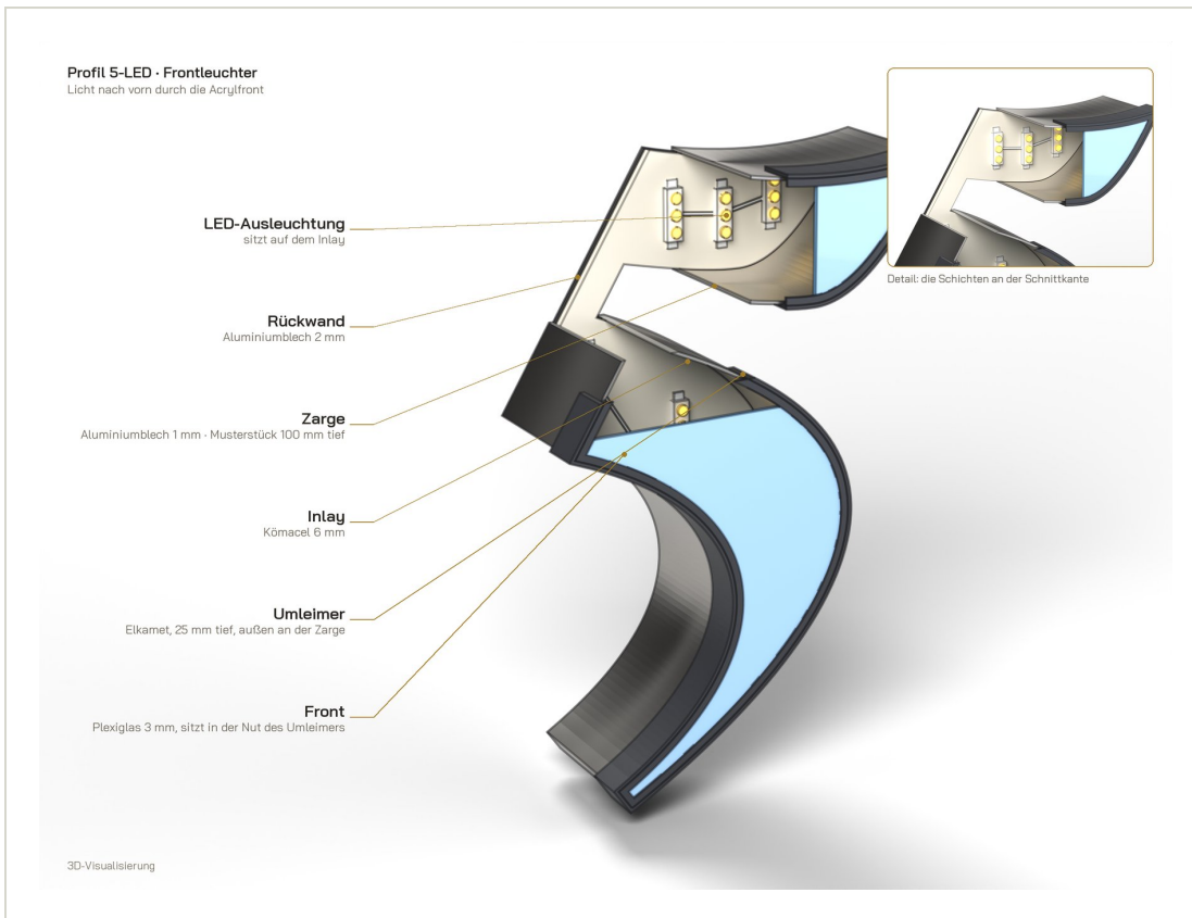
SCHNITT · PROFIL 5-LED
