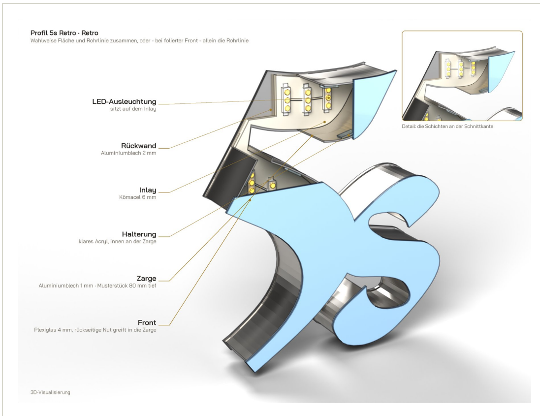
SCHNITT · PROFIL 5S RETRO
