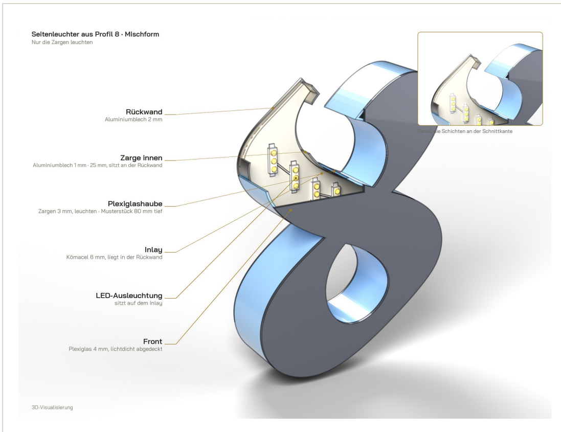
SCHNITT · SEITENLEUCHTER AUS PROFIL 8
